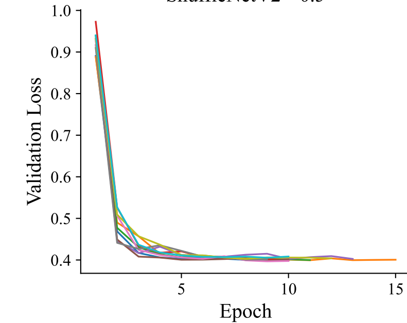
ShuffleNetV2- \times 0.5
