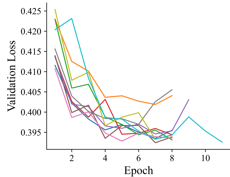
EfficientNet-B0
